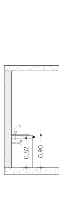
Bancada Pré-moldada em Betão a vista (dim=180x60x8cm)
