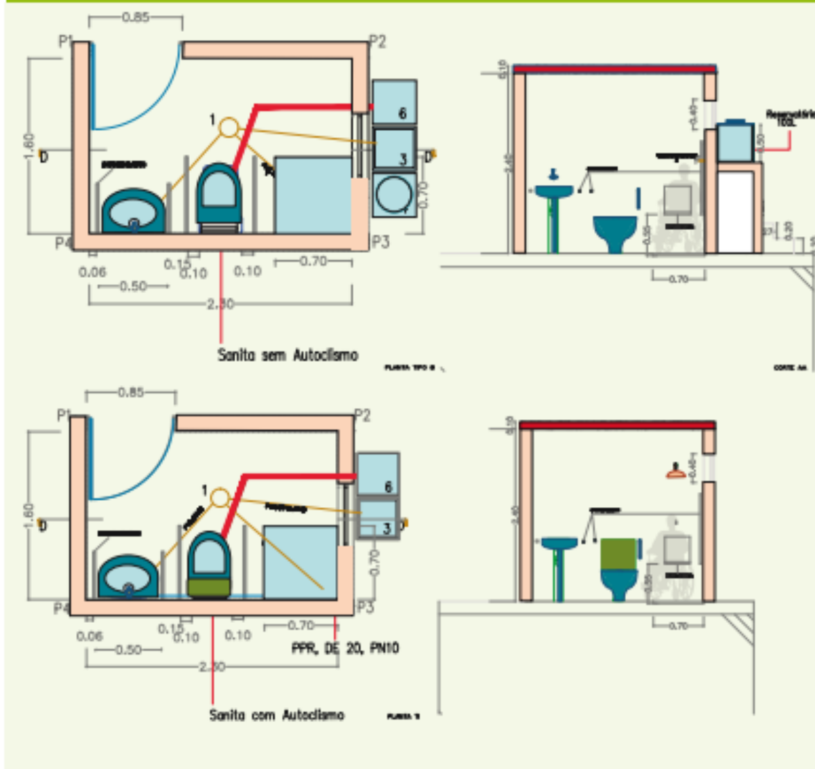
Figura 12. Instalação sanitária – Tipos C1 e C2
